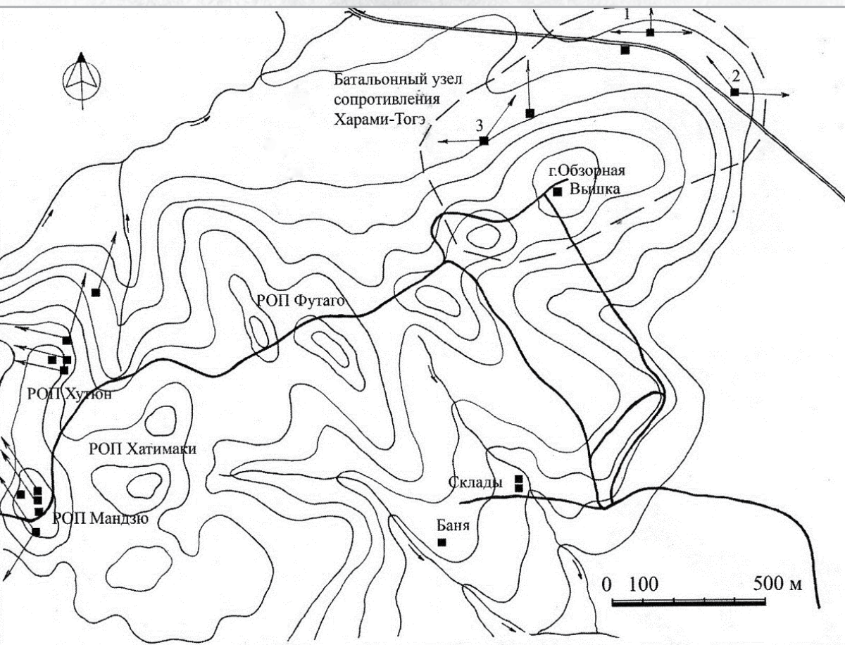
План батальонного узла сопротивления Харами-Тогэ (на схеме не обозначены три дота). И. Самарин «Сталь и бетон арафута», 2007 г., стр. 21
